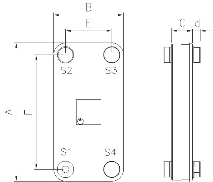
Scambiatore 180 kW
