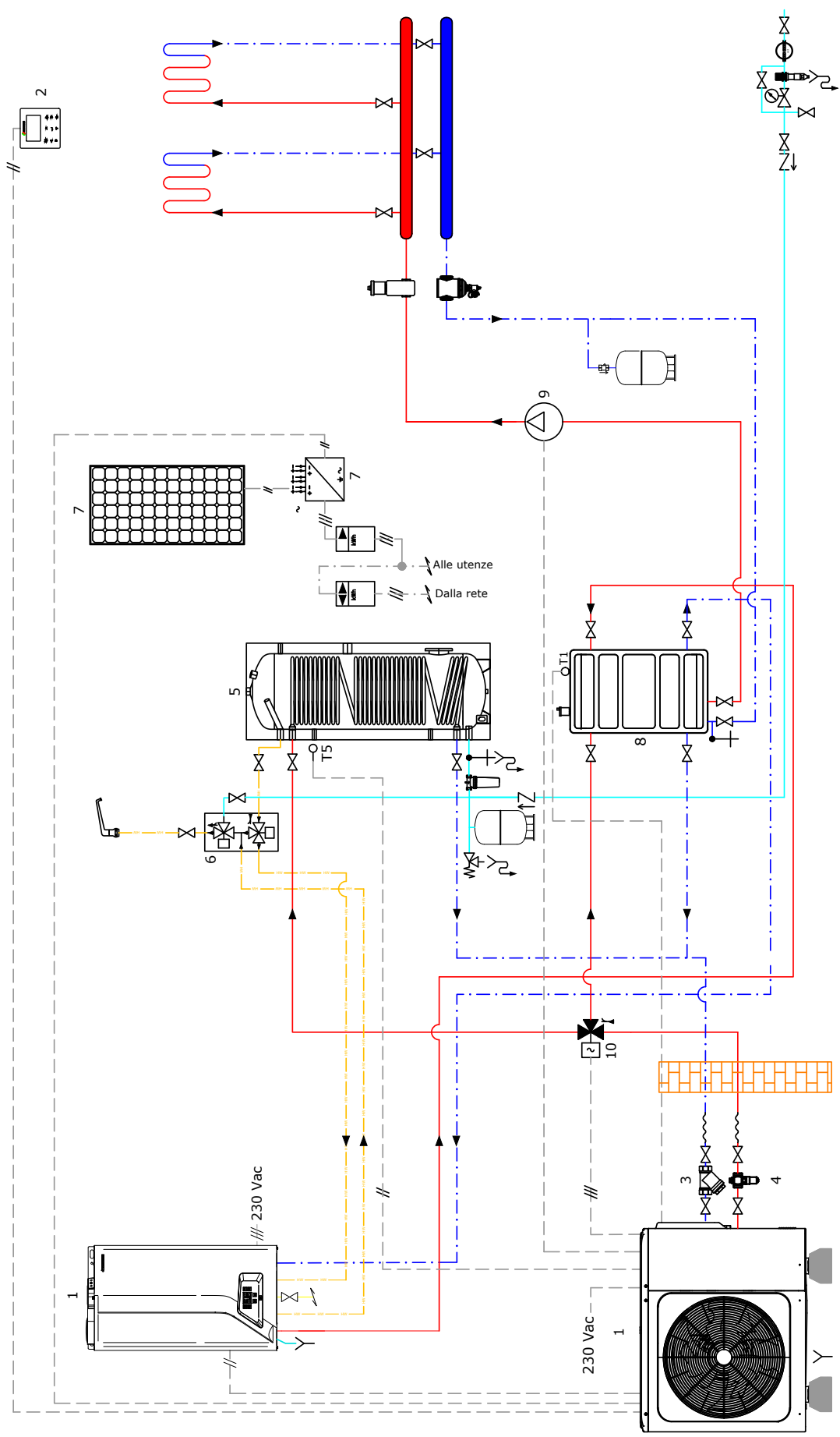
Schema di impianto indicativo e non sostitutivo di una progettazione tecnica.
