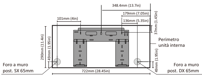
Clima Top 9 Mono (unità interna)
