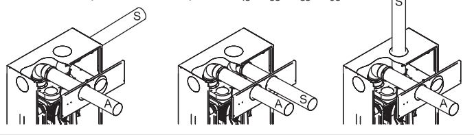
Esempi di sistemi con aspirazione diretta B 23
