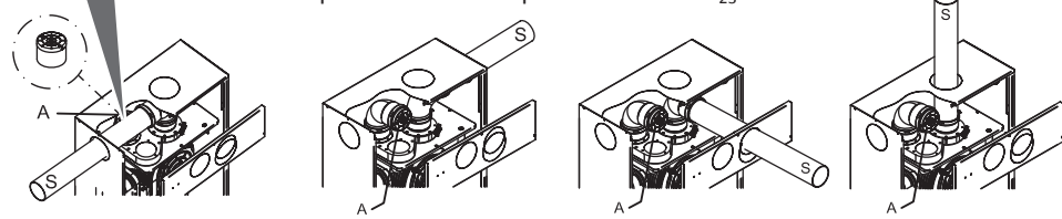
Esempi di sistemi con aspirazione diretta B_{23}
