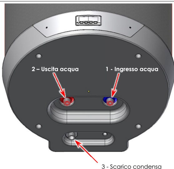
Fig. 7- Collegamento idrico
