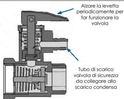
Fig. 8- Valvola di sicurezza 7 bar (0,7 MPa) per scaldabagno
