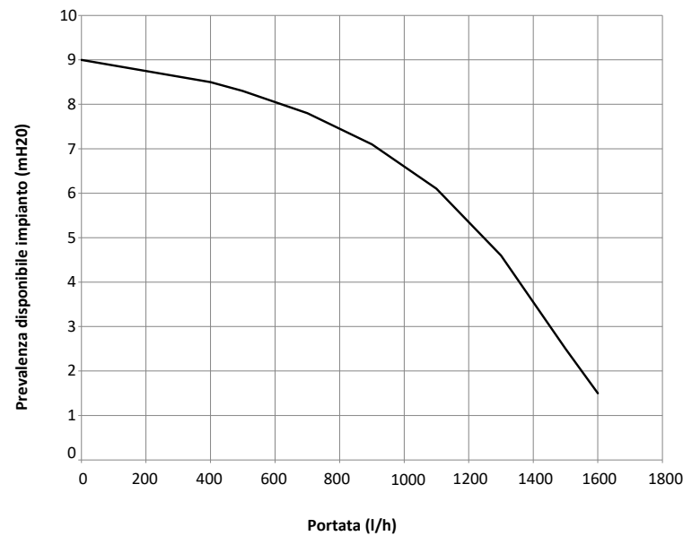
Curva di portata e prevalenza Top Energy circolatore supplementare zona miscelata UPM4XL 25-90
