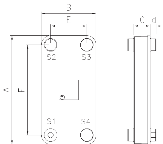
Scambiatore 180 kW
