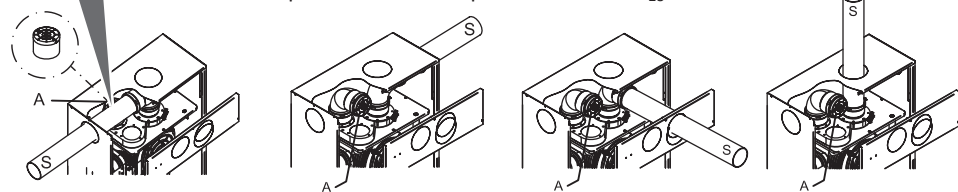
Esempi di sistemi con aspirazione diretta B_{23}
