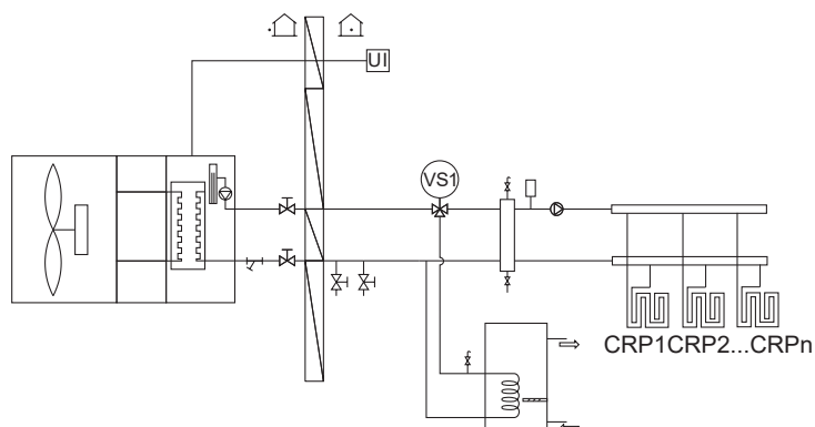
Schema dell'impianto 2
