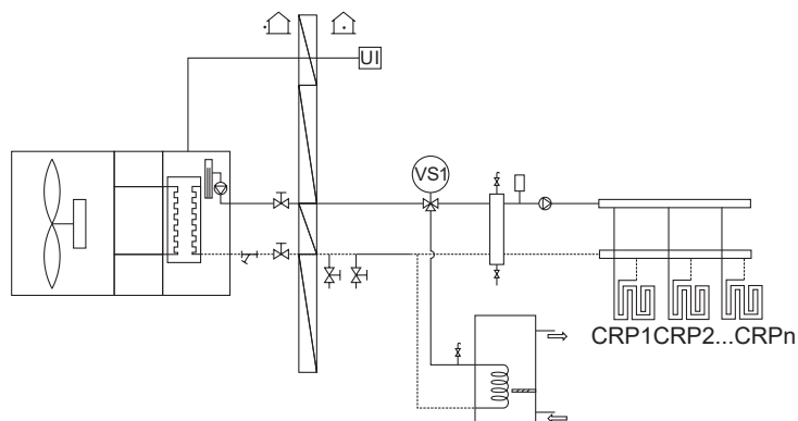
Schema dell'impianto 1
